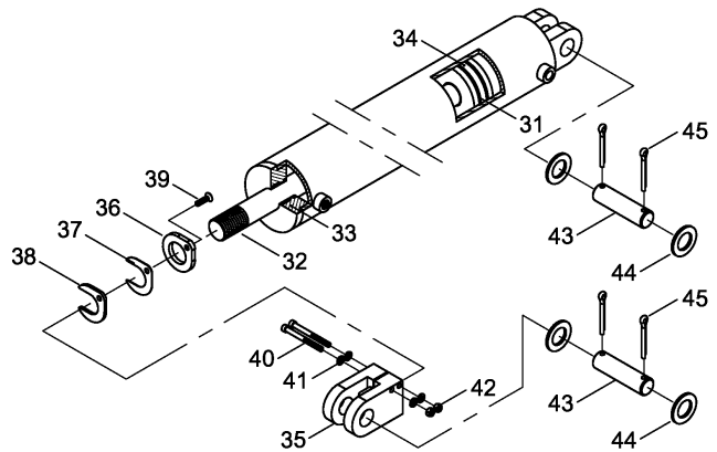
⑳ Hyd.- Zylinder DZ 100 x 40 x 715 00130370
